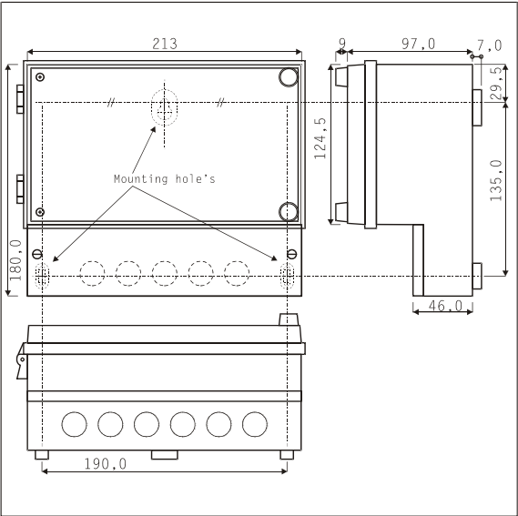
Behuizing zonder deur tek.940024
