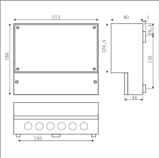
Behuizing met deur tek.941402
