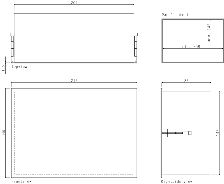
Maatgegevens inbouw behuizing tek. 961271
